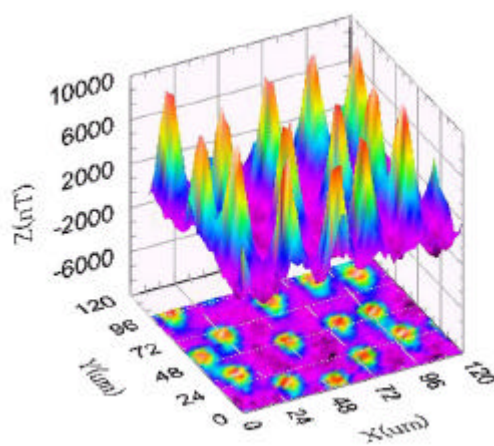
図 1 . 高温超伝導体 \text{YBa}_2\text{Cu}_3\text{O}_7 薄膜にトラップされた量子化磁束。各々は 2.07 \times 10^{-7} \text{ Gcm}^2 の値を持ち、この値以外のものは観測されない。
