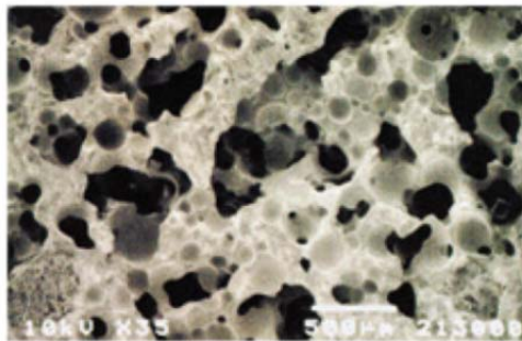
図 14.3 \beta - リン酸三カルシウム多孔体の気孔構造(オリンパス) (出典: セラミックス, 43 (2008) 987)
