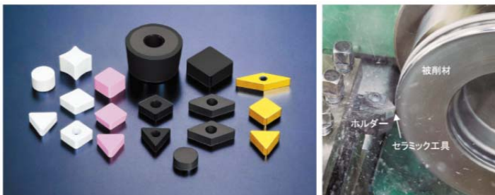
図 1.2 セラミック工具とホルダー (日本特殊陶業) (出典:セラミックス, 43 [8] 661 (2008).)
