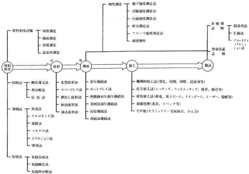
図 1.5 1980 年代前半の標準的ファインセラミックス製造プロセス (出典: ファインセラミックス基本問題懇談会報告書)
