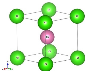
図 2.3 CsCl 構造 ( a=4.123 \text{ \AA} )
