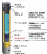
図 2.2 ナトリウム硫黄電池の単セル(日本ガイシ)。(出典:セラミックス, 42 [8] 613 (2007).)
